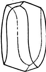
Calcite.
